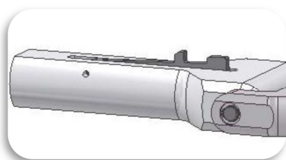
Braccio di reazione ad aggancio rapido con angolo variabile
