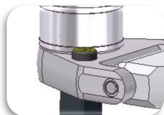
Livella integrata per una perfetta perpendicolarità
